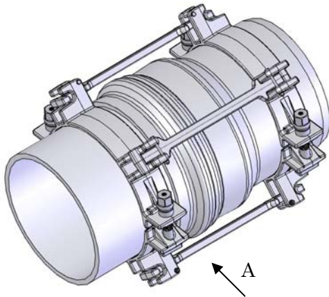
A矢視図
